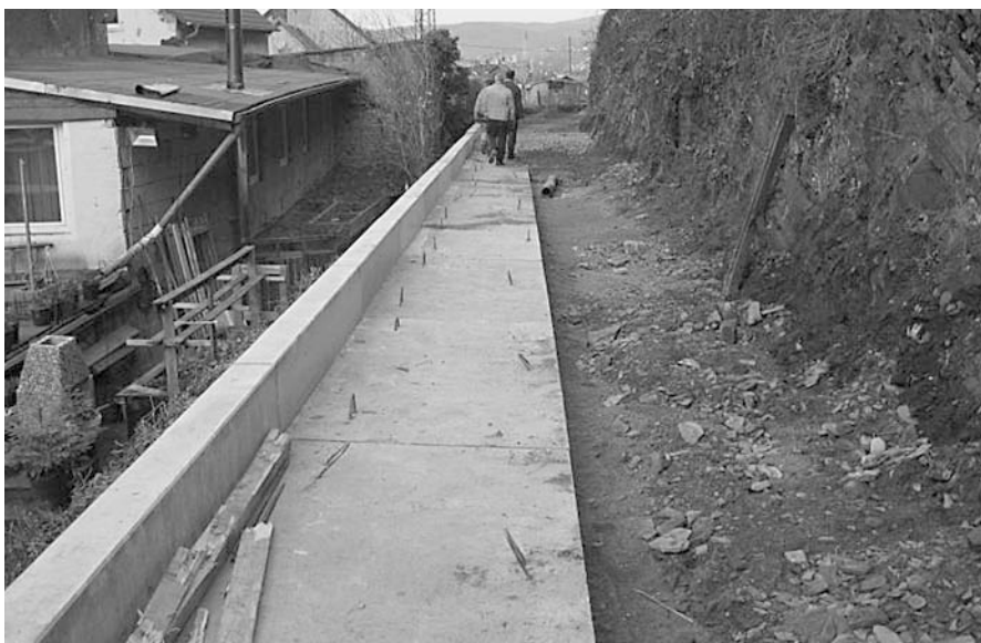
Montierte Winkelhalteplatten zur Schottersicherung.
